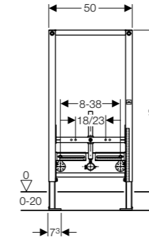
Geberit Duofix frame for bidet, 98cm, Universal
