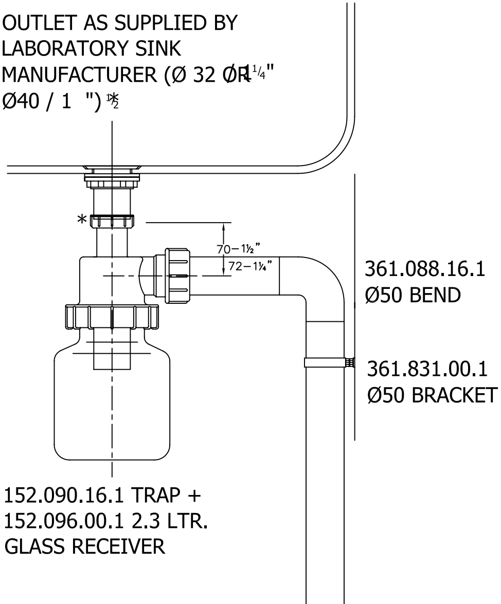
361.000.00.1 Ø50 PIPE
